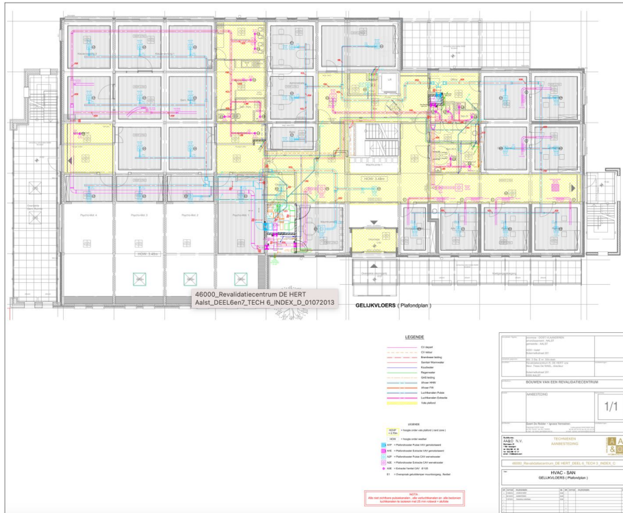
HVAC/SAN – Plafondplan - Gelijkvloers
