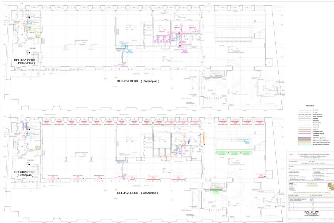
HVAC/SAN – Grond – en plafondplan - Gelijkvloers
